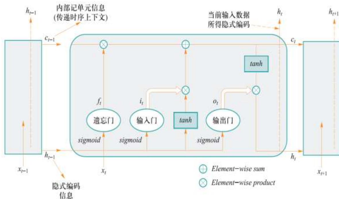
图 5.19 长短时记忆网络模型
