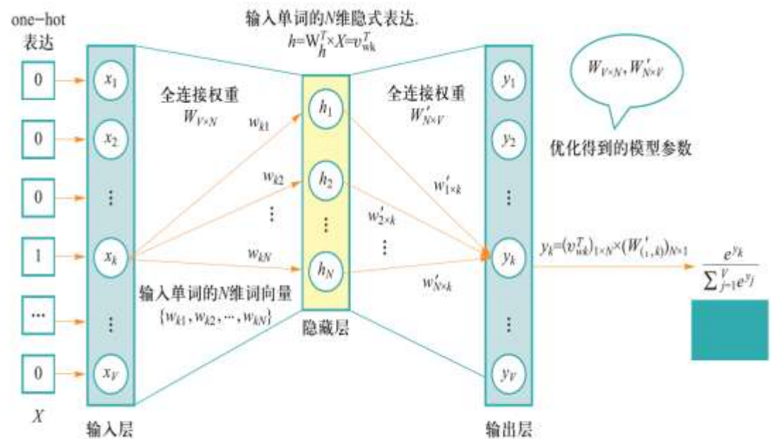
图 5.24 单个单词的词向量生成示意
