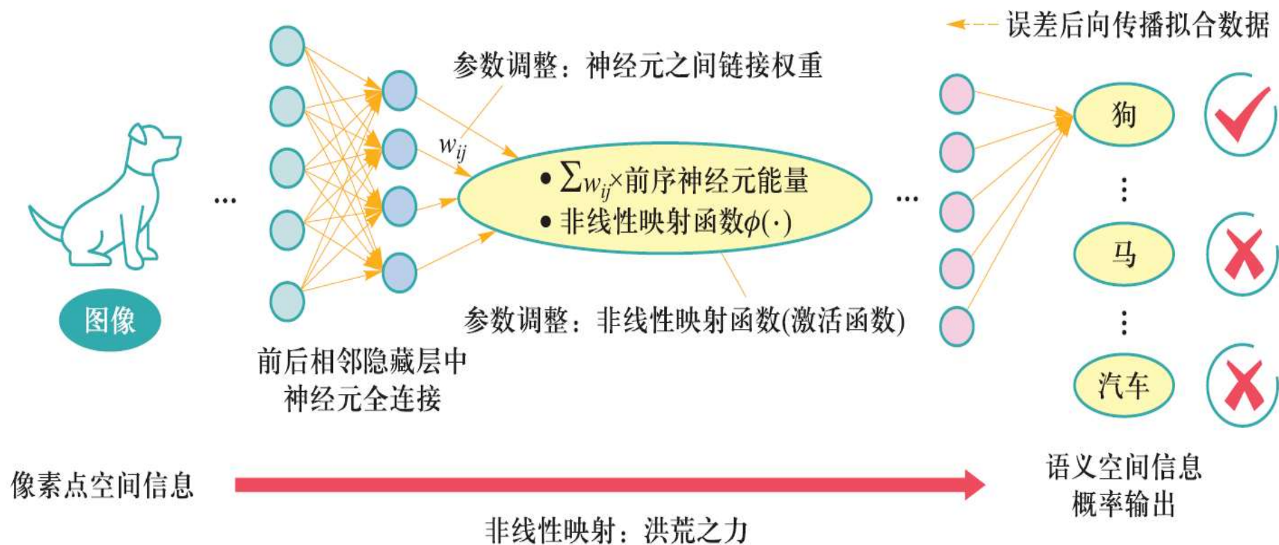
图 5.4 前馈神经网络模型
